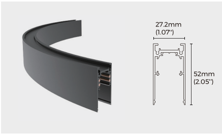
Ceiling / Pendant track
